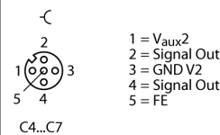
sortie M12 x 1
