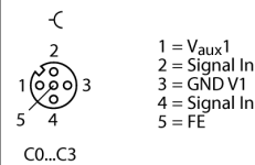
entrée M12 x 1
